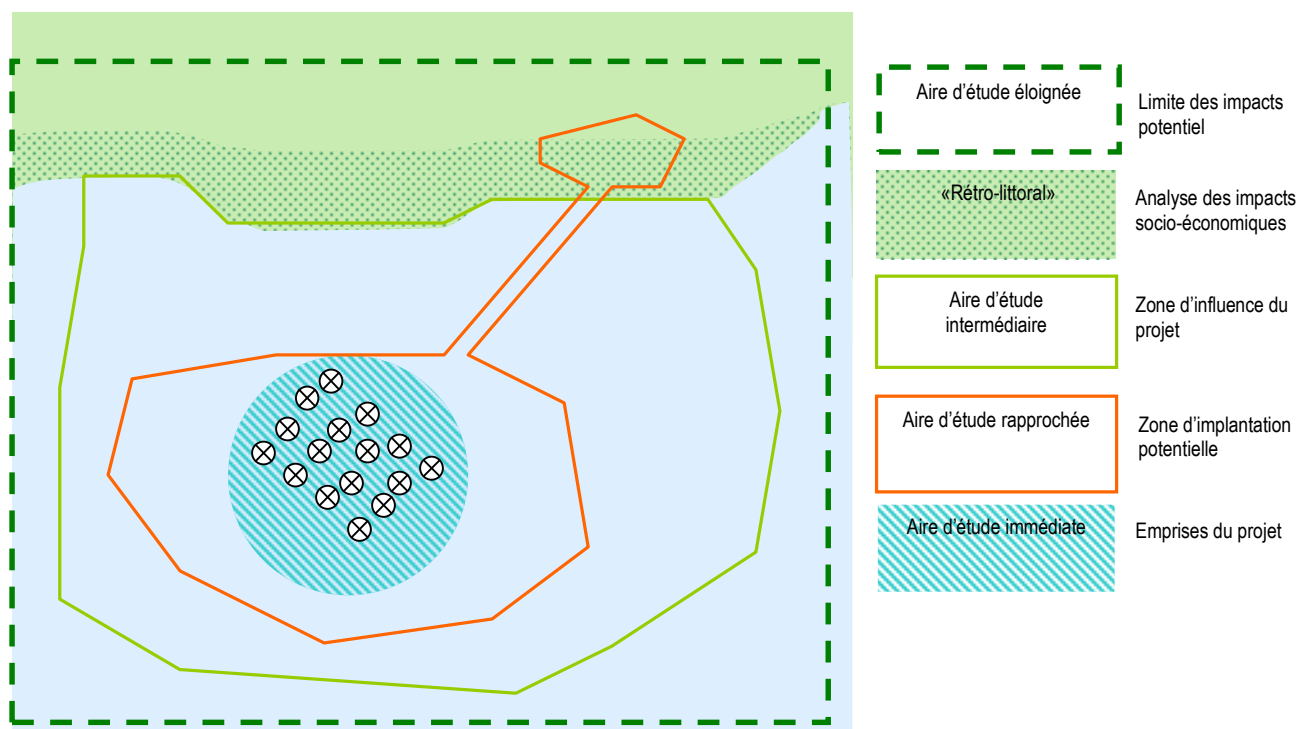
Figure 11 - Aires d'études pour un projet éolien en mer (échelle non représentative)
