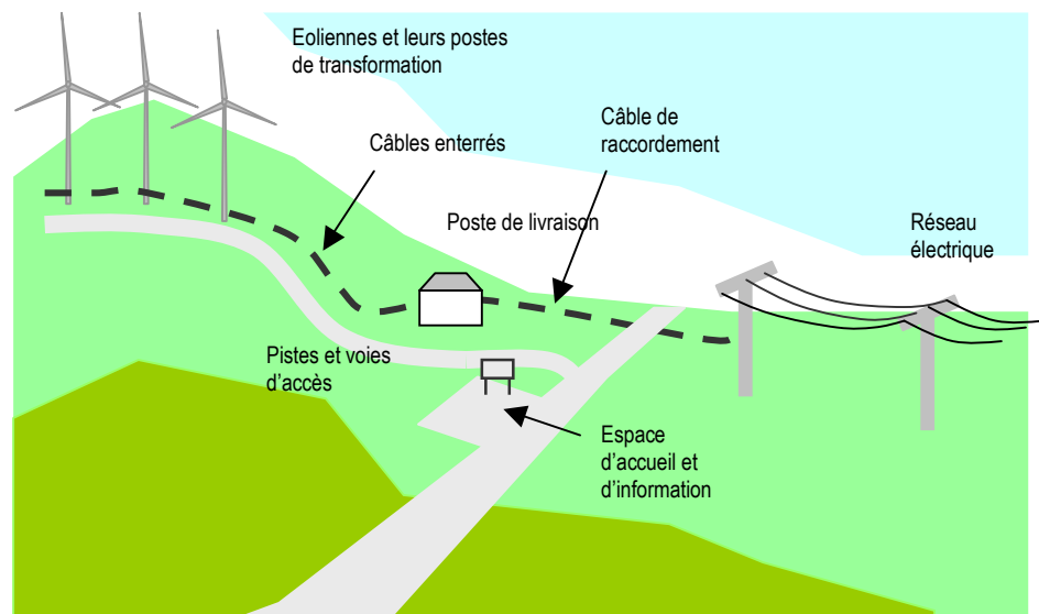
Figure 3 - Schéma descriptif d'un parc éolien terrestre (rapports d'échelle non représentatifs)
