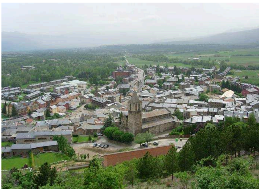
Figura 13.14: L'antiga capital de la Cerdanya, Llivia, i l'actual, Puigcerdà, es troben separades per escassos quilòmetres, tal i com s'aprecia en aquesta imatge presa des dels vessants del turó del castell de Llivia
