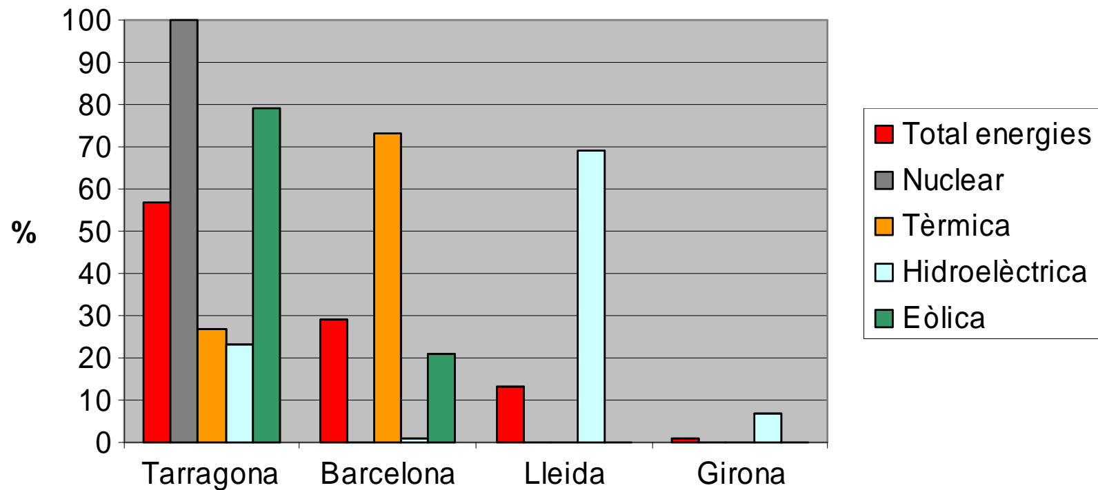
Potència elèctrica segons demarcació i tipus d'instal·lació (any 2005)
