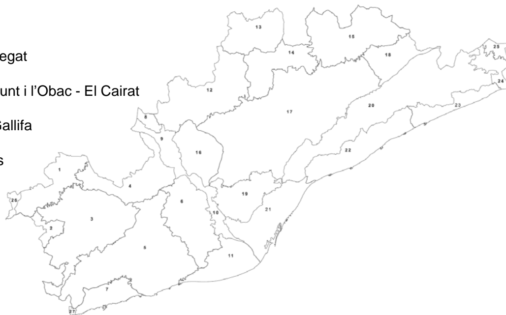
Figura 1: Esquema de les unitats de paisatge de la Regió Metropolitana de Barcelona.
